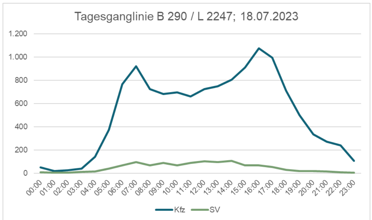
Abbildung 8: Tagesganglinie B 290 / L 2247 18.07.2023
