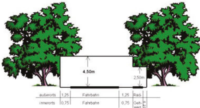
Lichtraumprofil
